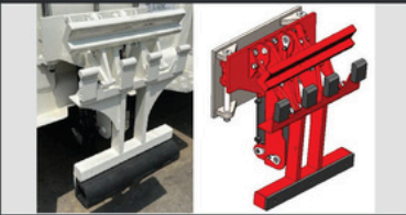
120/240/360 ltr bin lifter
